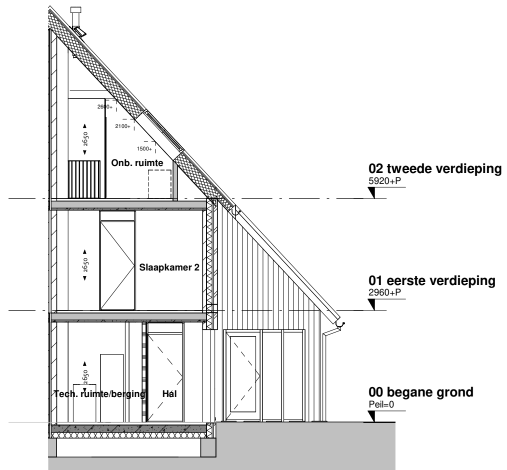
Doorsnede 1 : 100
