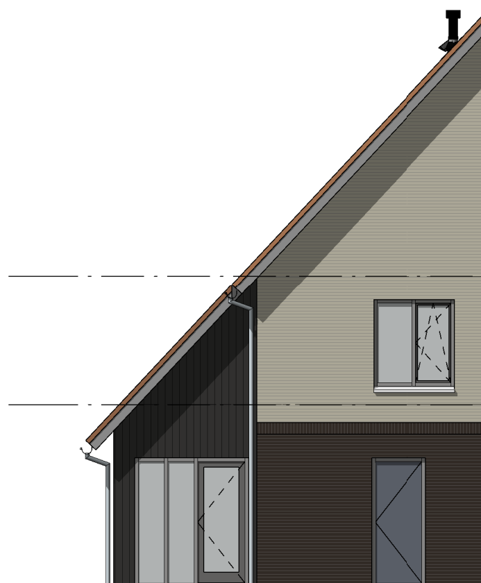
Zijaanzicht 1 : 100
