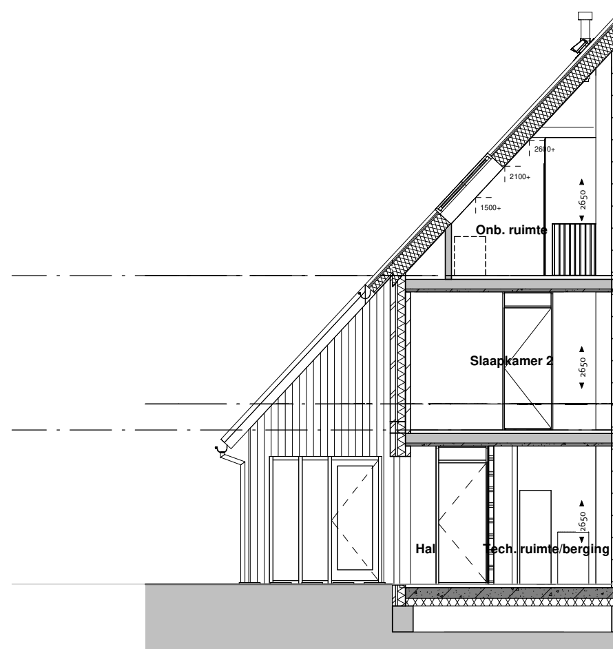
Doorsnede 1 : 100
